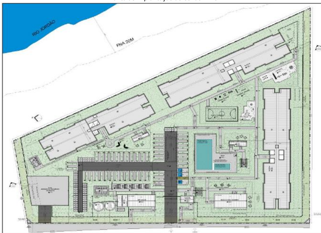
Planta de Implantação do Condomínio
