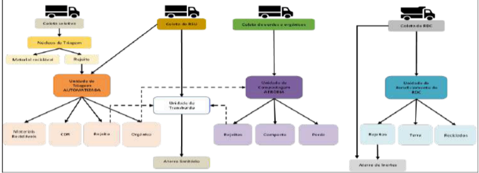
Figura 68: Fluxo da rota tecnológica do cenário referencial
